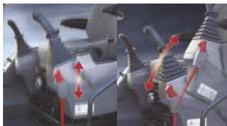
Bedieningspost (telescopische en kantelfunctie)
